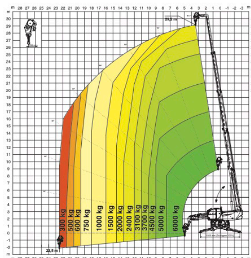
JIB CON ARGANO 1.500 kg
