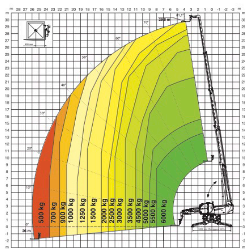
DIAGRAMMA PORTATE SU STABILIZZATORI ESTESI 360°
