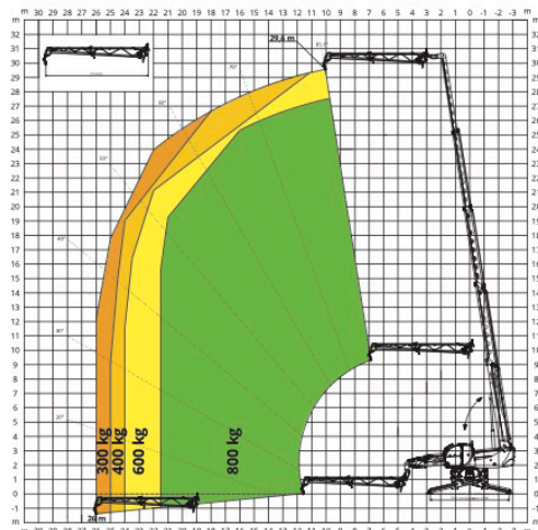
JIB CON ARGANO 800 kg
