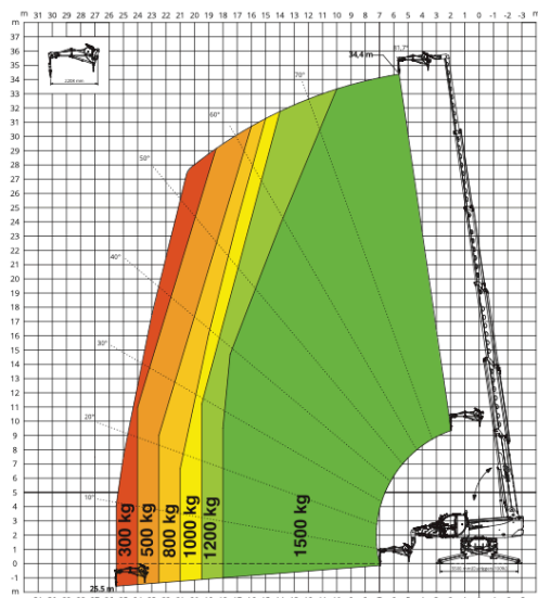
JIB CON ARGANO 1.500 kg
