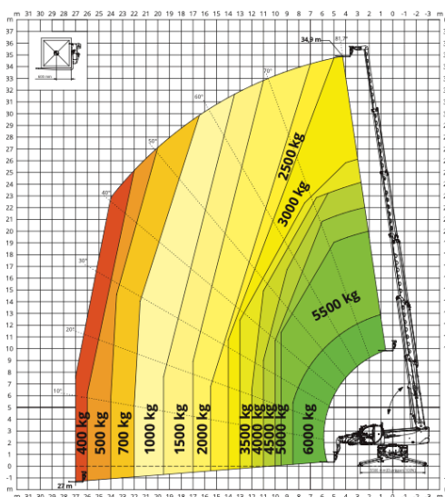
GANCIO 6.000 kg
