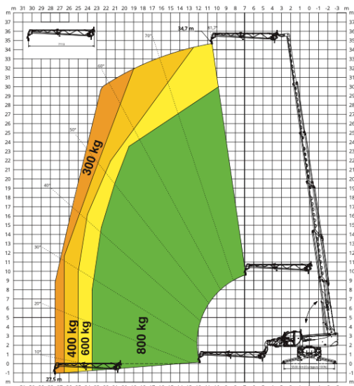
JIB CON ARGANO 800 kg
