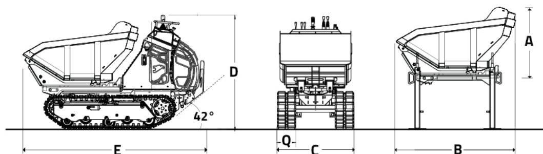
MACCHINA + ALLESTIMENTO
