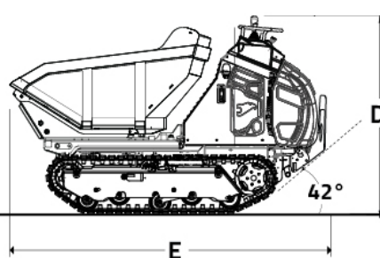
MACCHINA + ALLESTIMENTO
