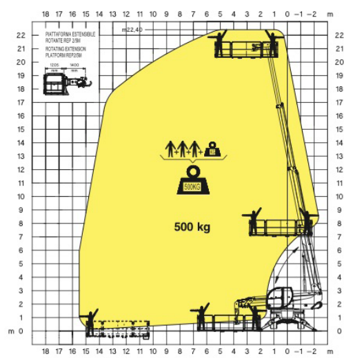
CESTELLO ESTENSIBILE ROTANTE 500 kg
