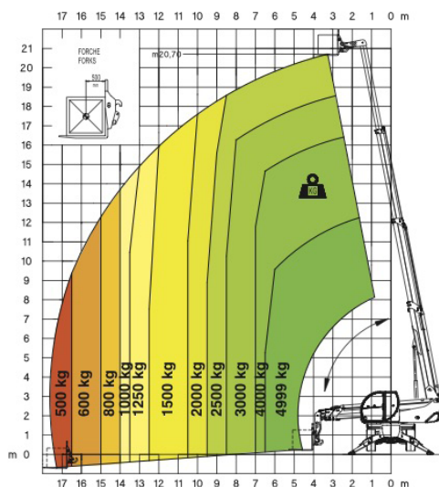
DIAGRAMMA PORTATE SU STABILIZZATORI ESTESI 360°
