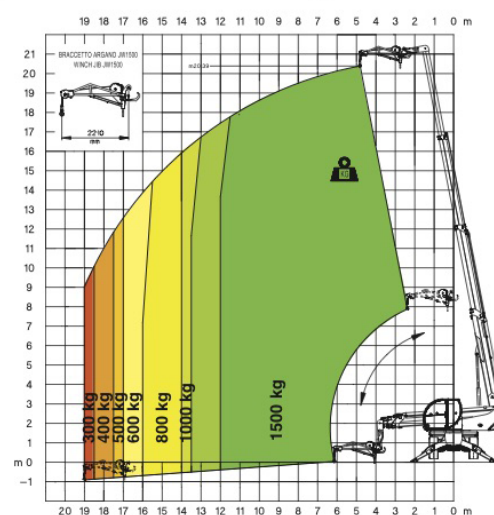
JIB CON ARGANO 1.500 kg
