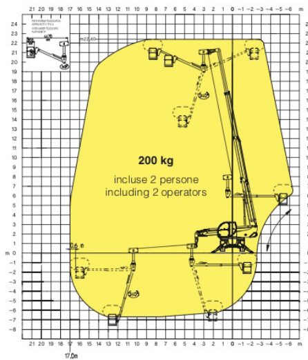
CESTELLO TELESCOPICO PIVOTANTE POSITIVO-NEGATIVO CON ROTAZIONE 340°
