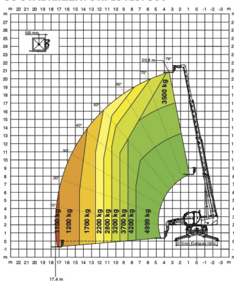
DIAGRAMMA PORTATE SU STABILIZZATORI ESTESI 360°
