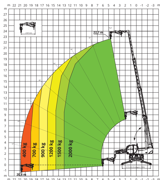
JIB CON ARGANO 2.000 kg
