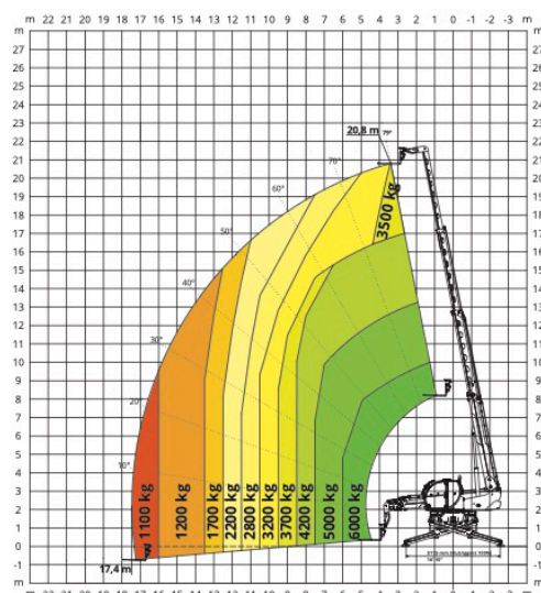
ARGANO 3.500 kg
